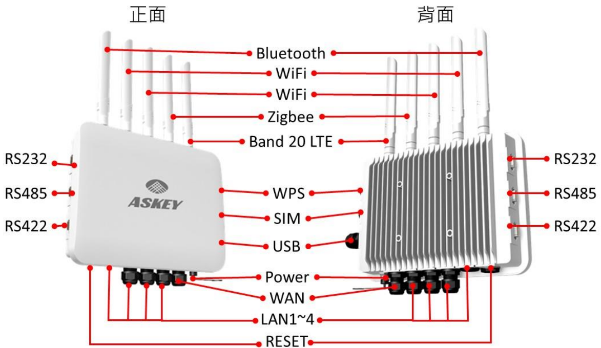
圖 2：物聯網開道器 APL2000W 外部介面
