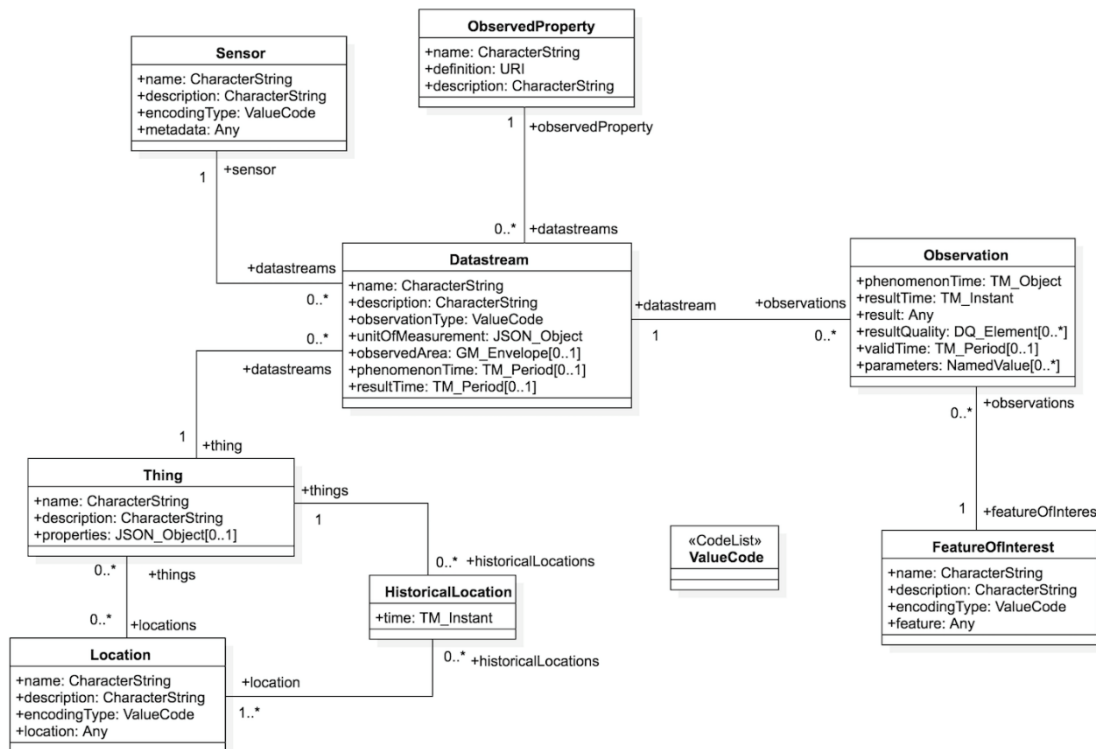
圖 1、SensorThings API 資料模型
