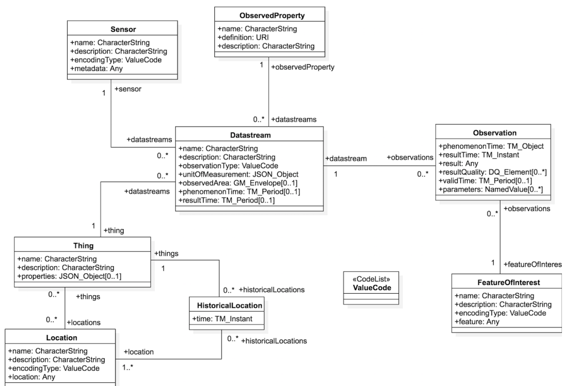
圖 1、SensorThings API 資料模型
